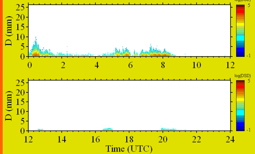
SVI DSD(m-3 mm-1). Hria: 2012/01/20. fmt(lin).
