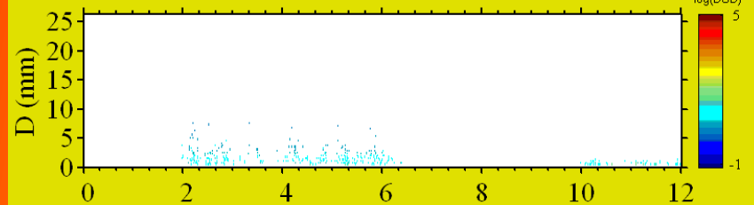
SVI DSD(m-3 mm-1). Hria: 2012/01/19. fmt(lin).
