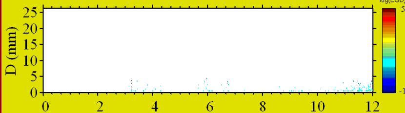
PVI DSD(m-3 mm-1). CarV: 2012/01/19. fmt(lin).
