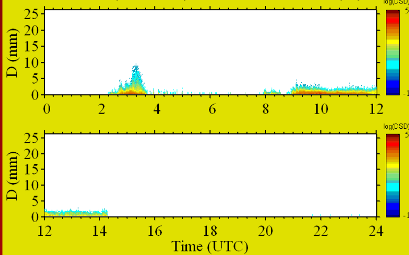
PVI DSD(m-3 mm-1). CarV: 2012/01/20. fmt(lin).
