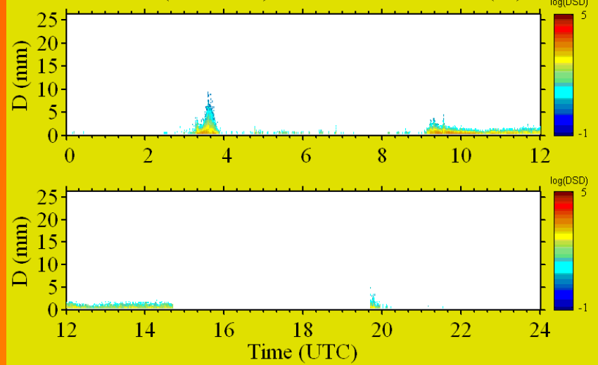
SVI DSD(m-3 mm-1). Smsw: 2012/01/20. fmt(lin).
