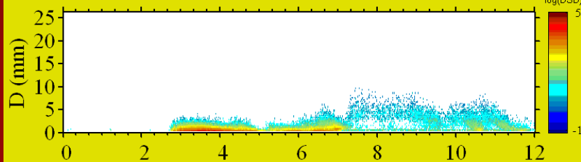
PVI DSD(m-3 mm-1). CarV: 2012/01/21. fmt(lin).
