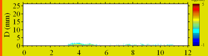
SVI DSD(m-3 mm-1). Hria: 2012/01/21. fmt(lin).
